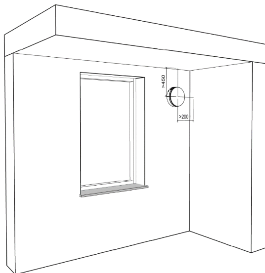
Figure 4 - Distances minimales par rapport aux éléments de construction (en mm)
