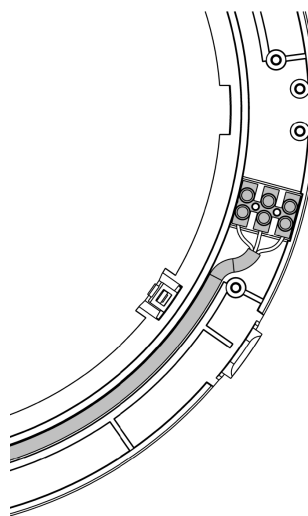
Figure 34 - Raccordez le câble interne à la borne 2.
