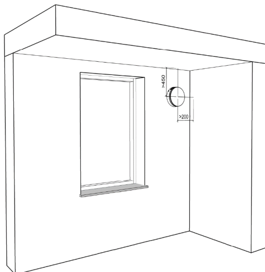
Figure 4 - Distances minimales par rapport aux éléments de construction (en mm)
