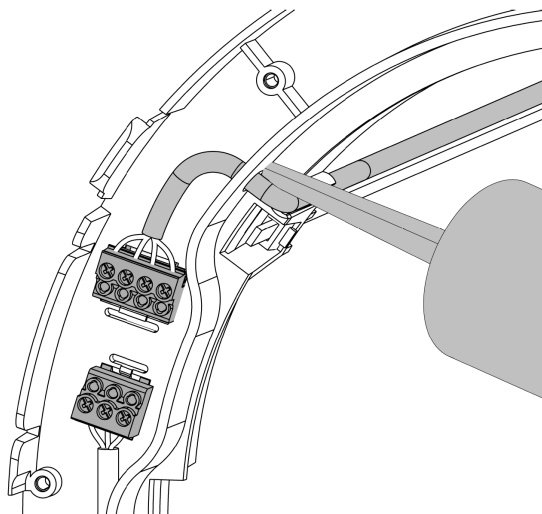
Figure 28 - Obturation du trou du câble
