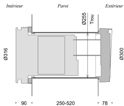
Figure 2 - Dimensions. Toutes les dimensions sont en [mm]
