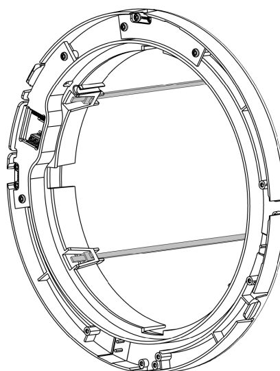
Figure 25 - Le chapeau de façade est désormais fixé.
