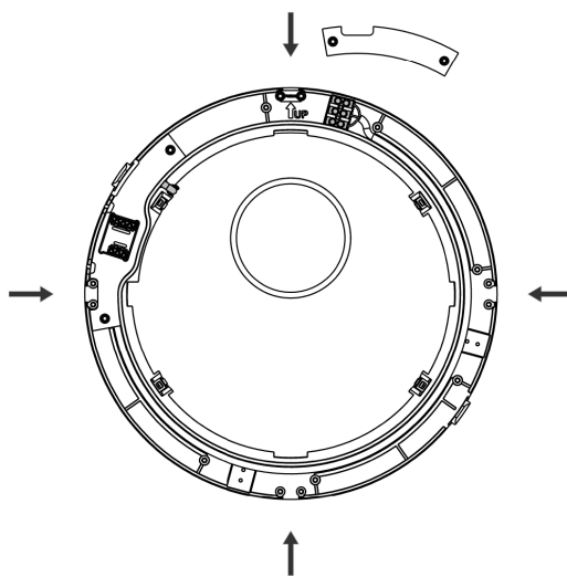
Figure 29 - Raccordement du câble de 230V ; plusieurs options possibles
