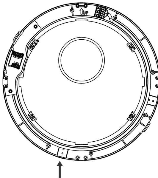
Figure 36 - Emplacement de la borne 2 en cas de passage des câbles par le bas
