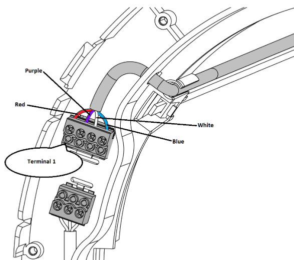
Figure 27 - Raccordement du câble de 24V à la borne 1
