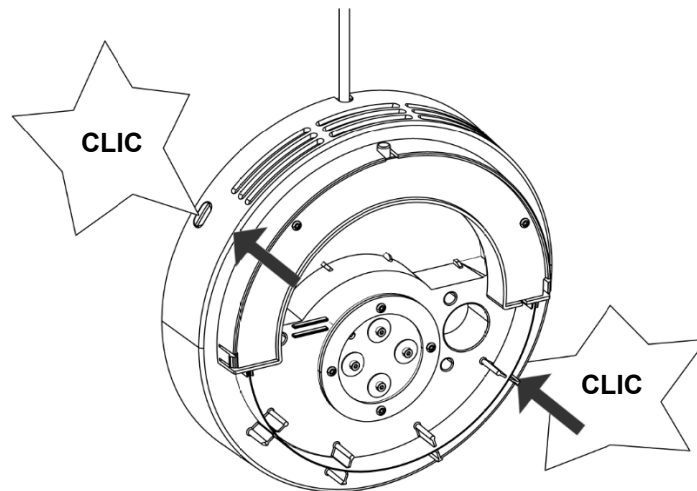
Figure 43 - Centrale insérée dans le chapeau de façade
