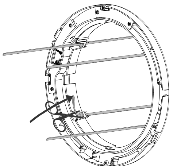
Figure 24 - Pliez et coupez les autres bandes.
