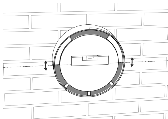
Figure 16 - Chapeau de ventilation de niveau
