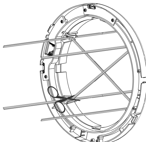
Figure 23 - Pliez et coupez les bandes « montées ».
