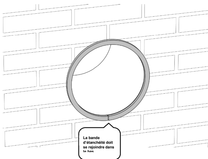
Figure 13 - Bande d'étanchéité extérieure
