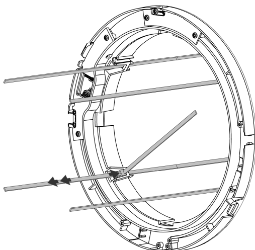
Figure 22 - Faites glisser les bandes.
