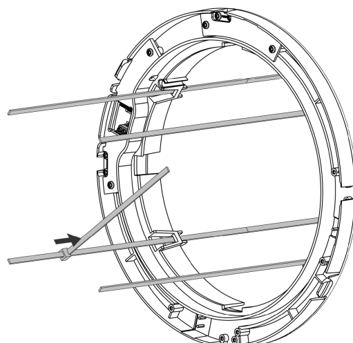
Figure 21 - Fixez une bande supplémentaire sur chaque bande.
