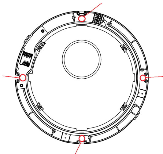
Figure 40 - Raccordement dissimulé du câble de 230V
