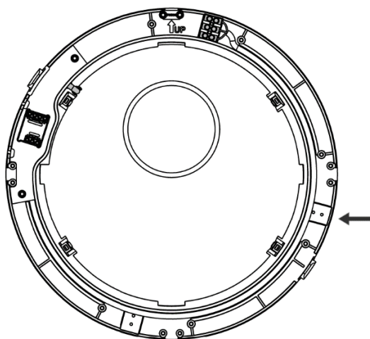
Figure 32 - Nouvel emplacement de la borne 2 en cas de raccordement du câble sur la droite
