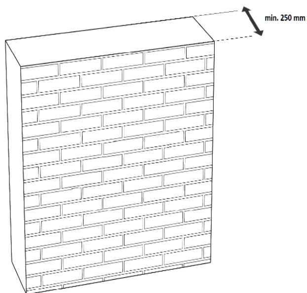
Figure 1 - Épaisseur de paroi minimale
