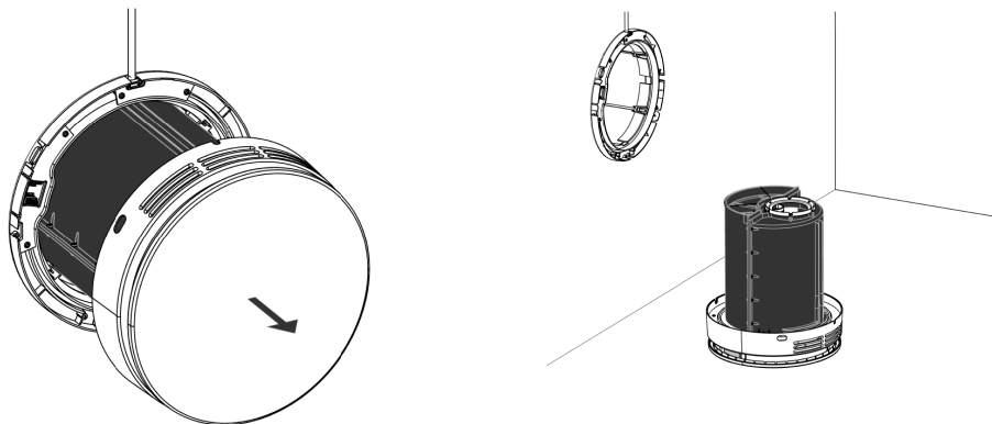
Figure 31 - Retirez la centrale et posez-la sur le couvercle intérieur.
