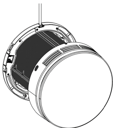
Figure 4 - Unité de ventilation à moitié sortie du support mural
