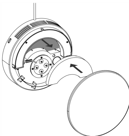
Figure 21 - Remplacez le filtre interne.
