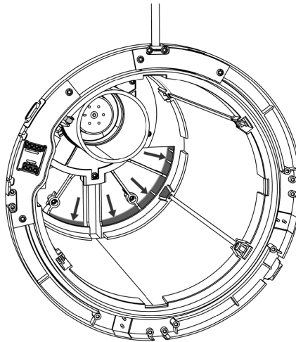
Figure 16 - Aspirez soigneusement le trou dans le mur ainsi que le filtre grossier situé à l'arrière.
