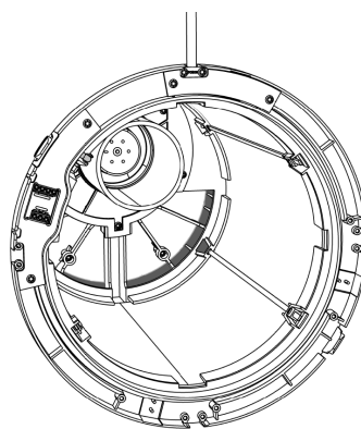
Figure 5 - Support mural et partie extérieure
