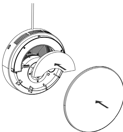
Figure 36 - Placez un nouveau filtre interne dans la centrale.
