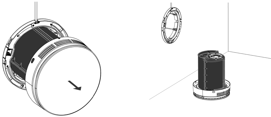
Figure 15 - Retirez la centrale et posez-la sur le couvercle intérieur.
