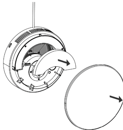
Figure 29 - Retirez le filtre interne.
