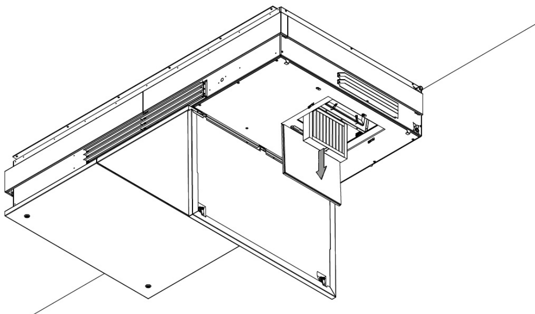
Illustration 15 : Retirer le filtre fin
