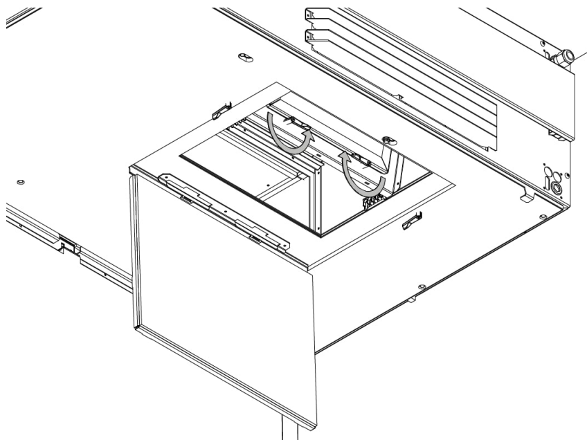
Illustration 13 : Fermer les charnières du filtre grossier
