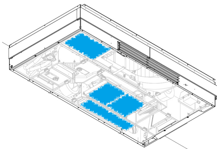
Illustration 22 : Emplacement du système de condensats dans la centrale AMX
