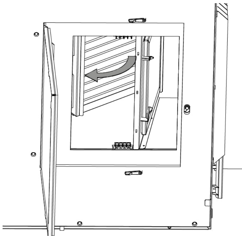
Illustration 14 : Ouvrir la charnière qui maintient le filtre fin en place
