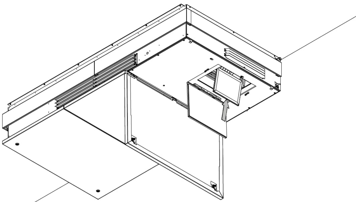
Illustration 12 : Remplacer le filtre grossier usagé par un filtre neuf
