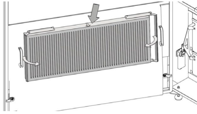
Filtre de la porte de service (filtre air repris)
