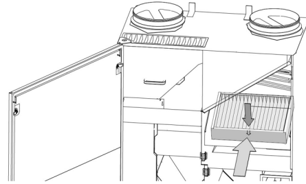
Filtre intérieur (filtre air frais)
